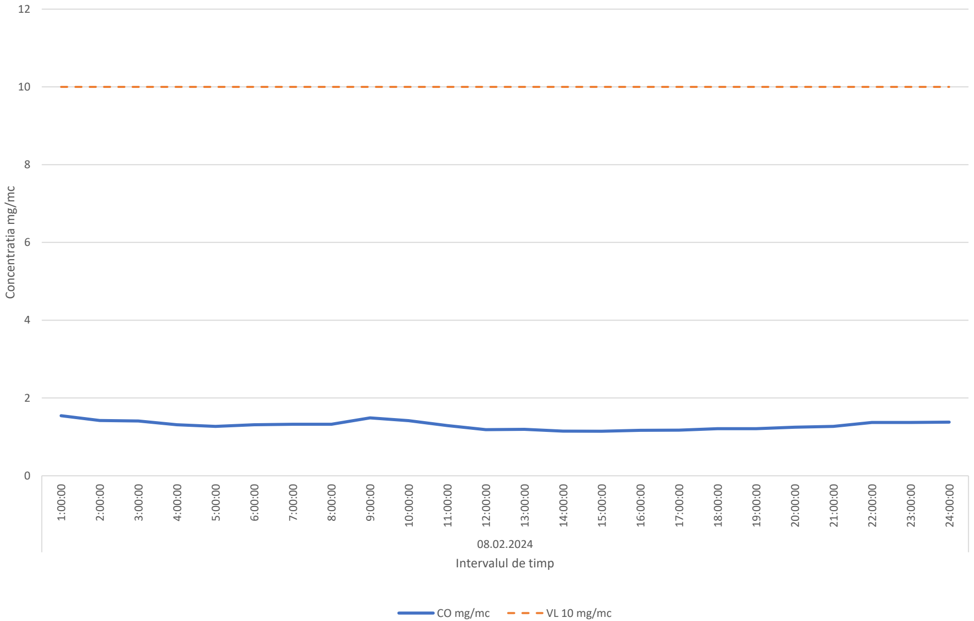
Variatia mediilor orare ale indicatorului CO in data de 08.02.2024 - Parcul Central, Municipiul Ploiesti
